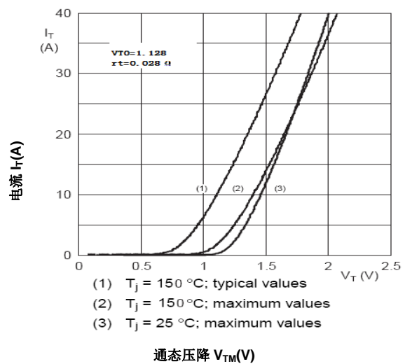
V_{TM} - I_T
