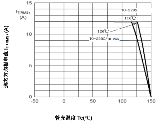
I_T(RMS) - T_c
