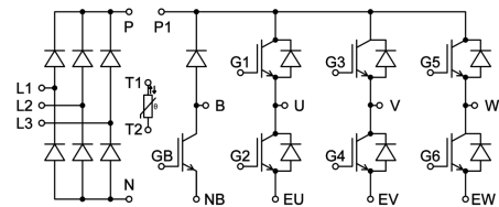
电路示意图
