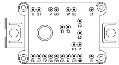
引脚示意图
